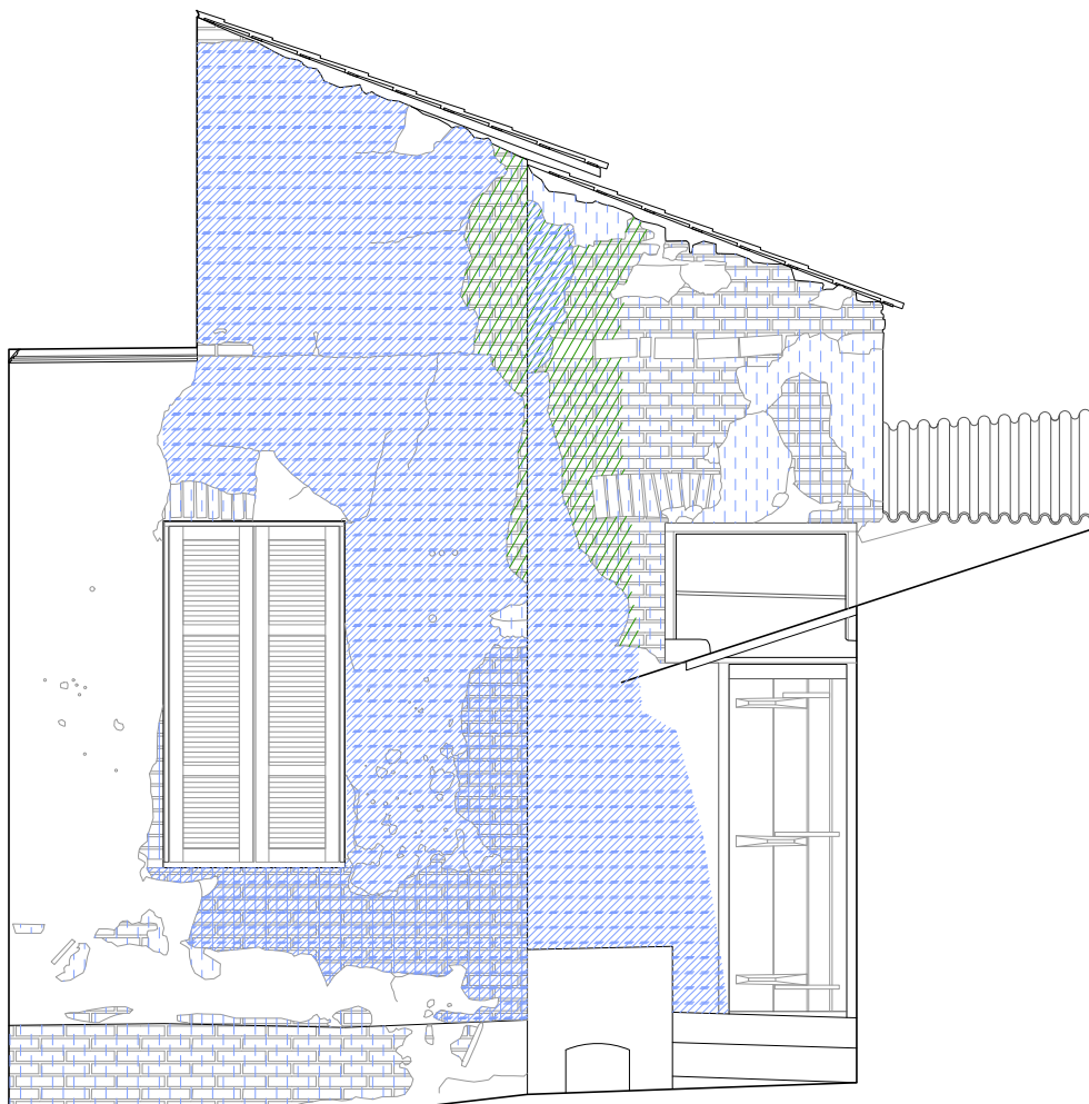
ELEVAÇÃO 8 | MAPEAMENTO DE DANOS ESCALA 1:50
