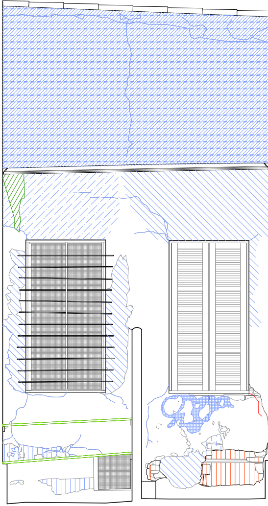
ELEVAÇÃO 7 | MAPEAMENTO DE DANOS ESCALA 1:50
