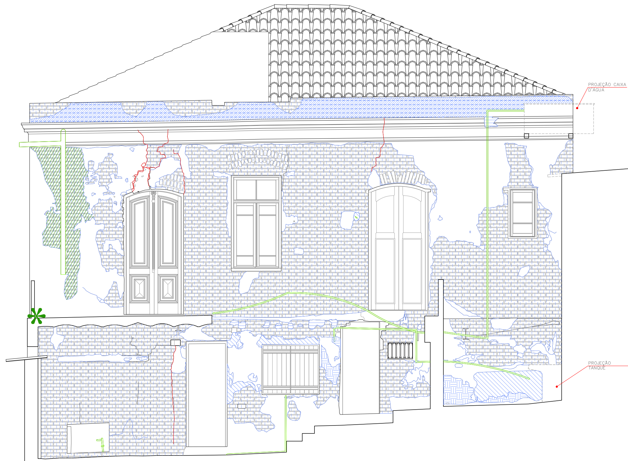
ELEVAÇÃO 02 | MAPEAMENTO DE DANOS ESCALA 1:50
