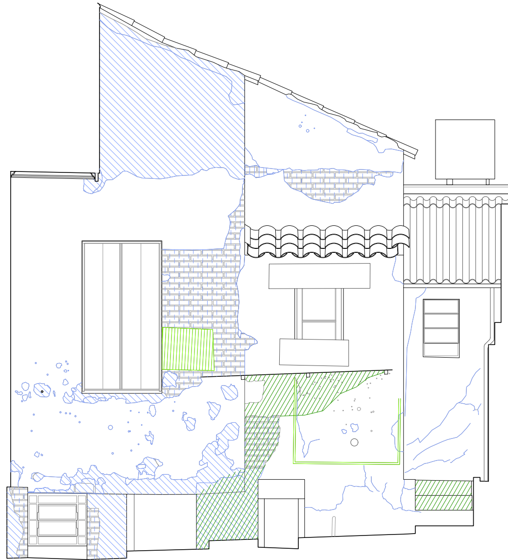
ELEVAÇÃO 5 | MAPEAMENTO DE DANOS ESCALA 1:50
