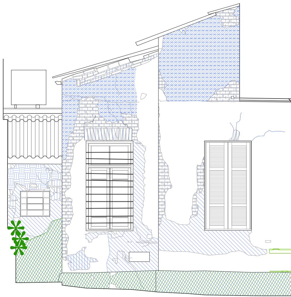
ELEVAÇÃO 6 | MAPEAMENTO DE DANOS ESCALA 1:50
