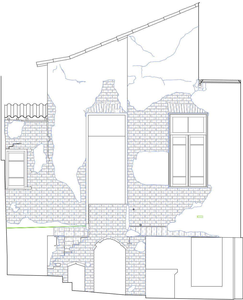
ELEVAÇÃO 3 | MAPEAMENTO DE DANOS ESCALA 1:50
