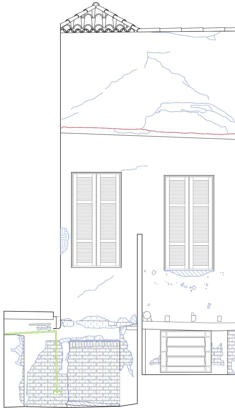
ELEVAÇÃO 4 | MAPEAMENTO DE DANOS ESCALA 1:50
