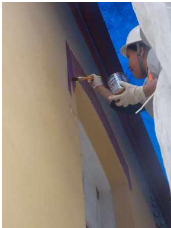
Foto 17 – Pintura lisa dos tijolos fingidos e molduras da fachada – Casa 06
