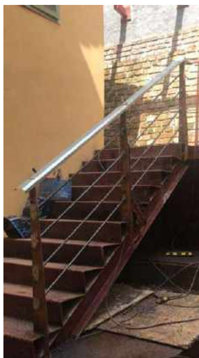
Foto 22 – Instalação do guarda corpo – Casa 06
