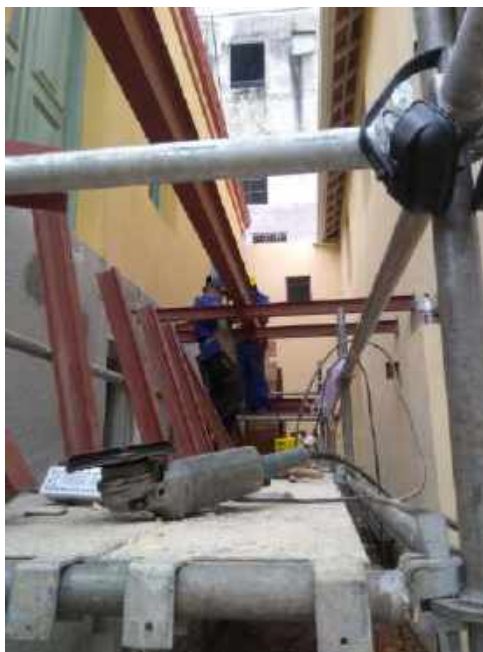
Foto 05 – Instalação dos ferros metálicos para execução da escada de alvenaria- Casa 06
